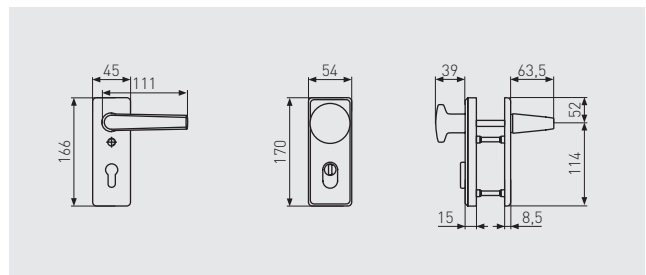
SCHUTZBESCHLAG HLT612
