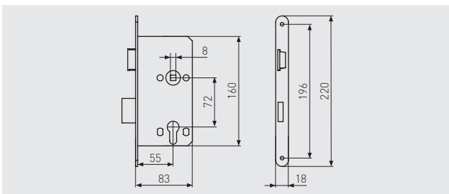
EINSTECKSCHLOSS FÜR WOHNUNGS- ABSCHLUSSTÜREN ES TGL PZ TGL-NORM
