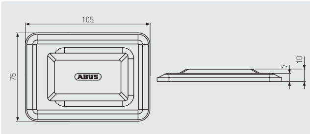
GITTERROSTSICHERUNG GS20
