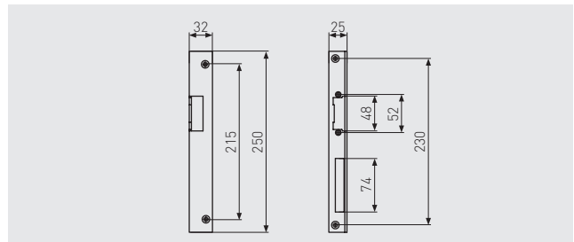
SCHLISSBLECH SB
