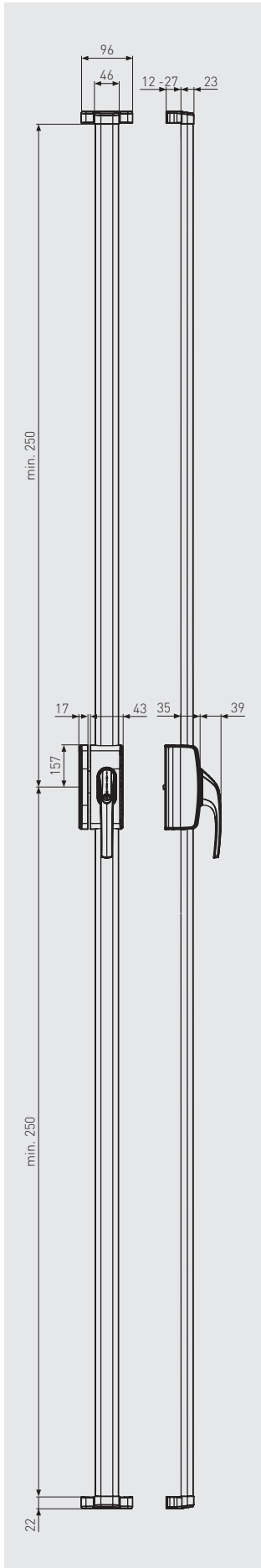
FENSTER-STANGENSCHLOSS FOS650
