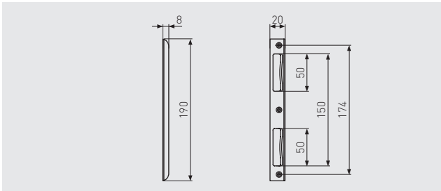
SICHERHEITS-WINKELSCHLISSBLECH FÜR HAUSTÜREN SSB400
