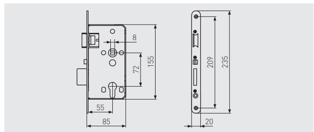
EINSTECKSCHLOSS FÜR WOHNUNGS- ABSCHLUSSTÜREN TKZ40
