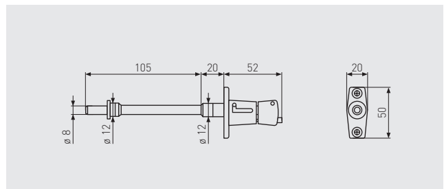
ROLLADENSICHERUNG RS87
