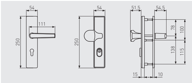
SCHUTZBESCHLAG KLZS714 ECKIG
