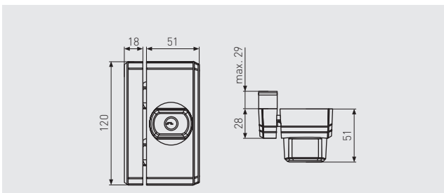
FENSTER-ZUSATZSICHERUNG FTS96
