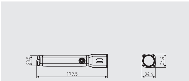
TASCHENLAMPE TL-517
