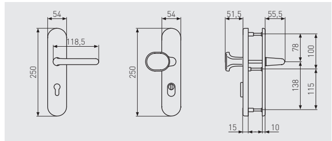
SCHUTZBESCHLAG KKZS700
