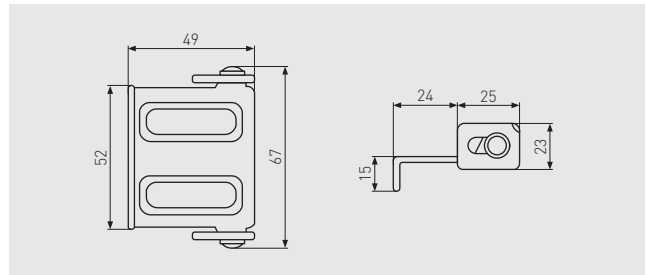
BALKONTÜRHEBEL-SICHERUNG BS84
