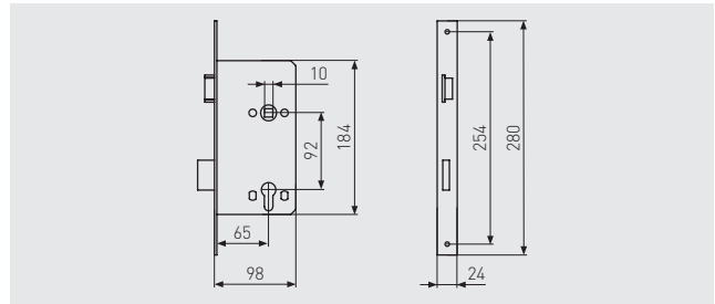
EINSTECKSCHLOSS FÜR WOHNUNGS- ABSCHLUSSTÜREN ES PZ2 RUNDER STULP
