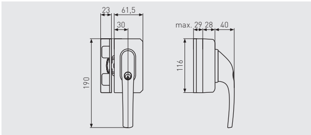
FENSTER-ZUSATZSICHERUNG F0400N
