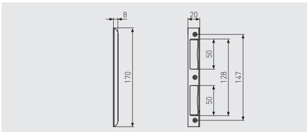
WINKELSCHLISSBLECH WST
