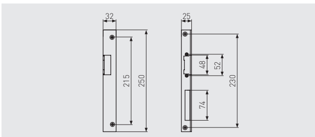
WINKELSCHLISSBLECH WST
