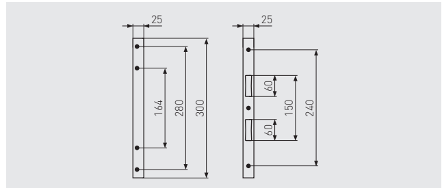
WINKELSCHLISSBLECH WSB170
