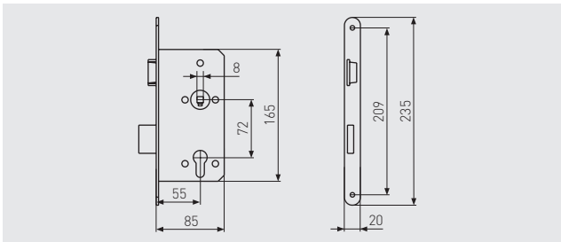
EINSTECKSCHLOSS FÜR WOHNUNGS- ABSCHLUSSTÜREN ES PZ2 KÄNTIGER STULP
