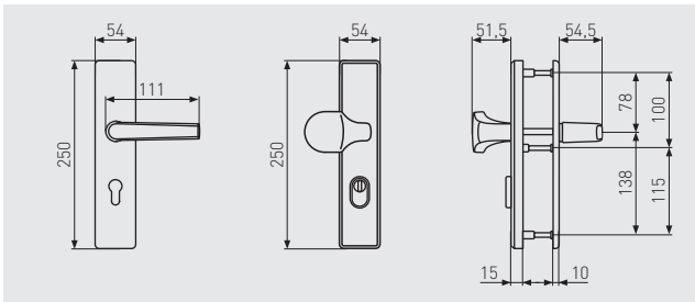
SCHUTZBESCHLAG KLZS714 FS
