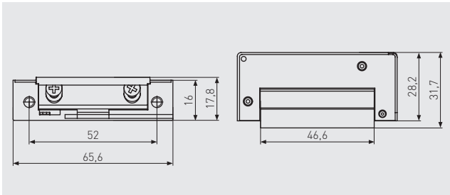
ELEKTRISCHER TÜRÖFFNER ET80
