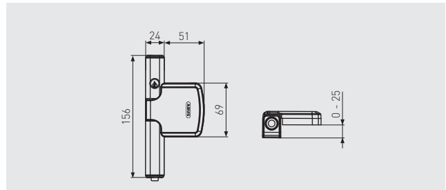
FENSTER-ZUSATZSICHERUNG MIT ALARM FTS96A
