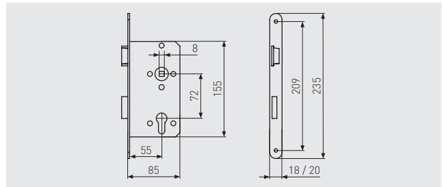
EINSTECKSCHLOSS FÜR WOHNUNGS- ABSCHLUSSTÜREN ESK PZ2 UNIVERSAL
