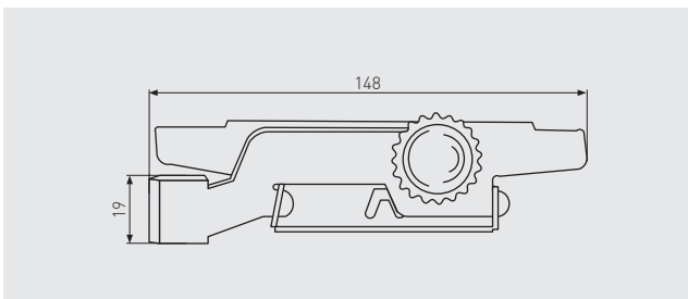
ROLLADENSICHERUNG RS97
