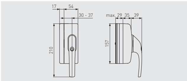
FENSTER-ZUSATZSICHERUNG FTS106
