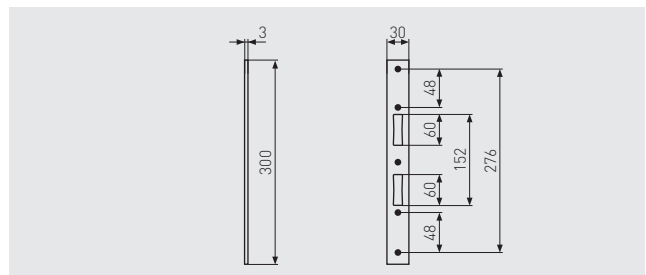
SCHLISSBLECH SB
