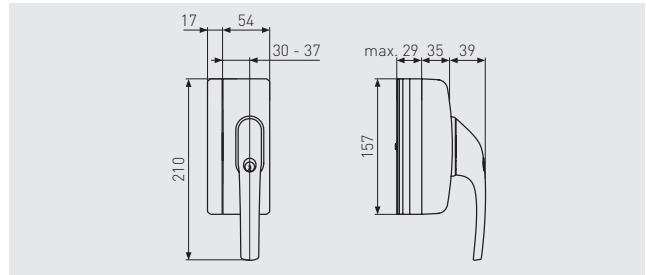
FENSTER-ZUSATZSICHERUNG FTS206
