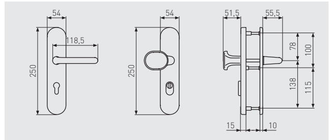
SCHUTZBESCHLAG KLZS714 RUND
