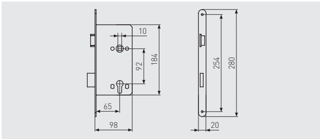
EINSTECKSCHLOSS FÜR WOHNUNGS- ABSCHLUSSTÜREN ES PZ3
